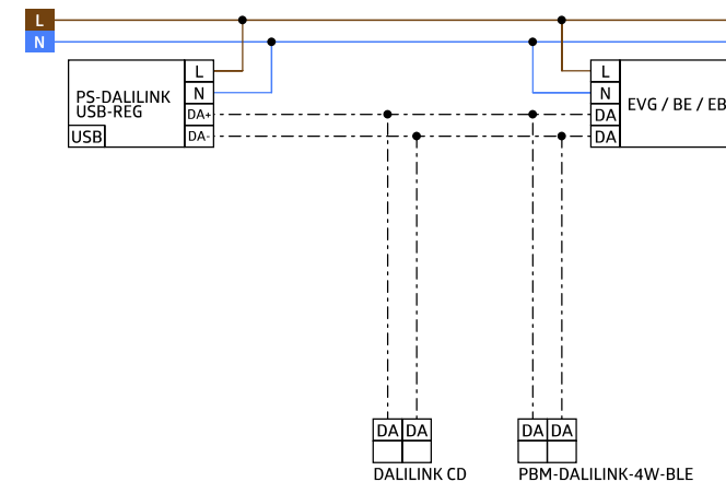
Schaltbild
