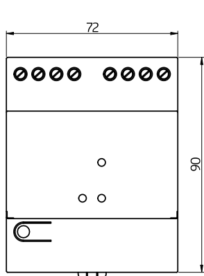
Bemaßung 93189
