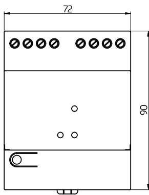
Bemaßung 93189
