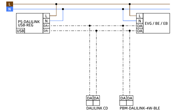
Schaltbild
