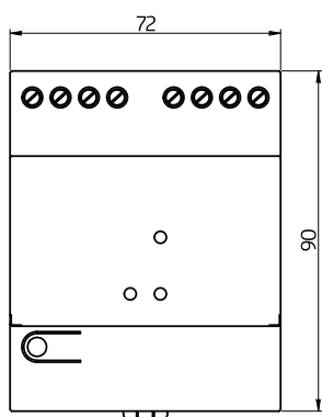
Bemaßung 93189
